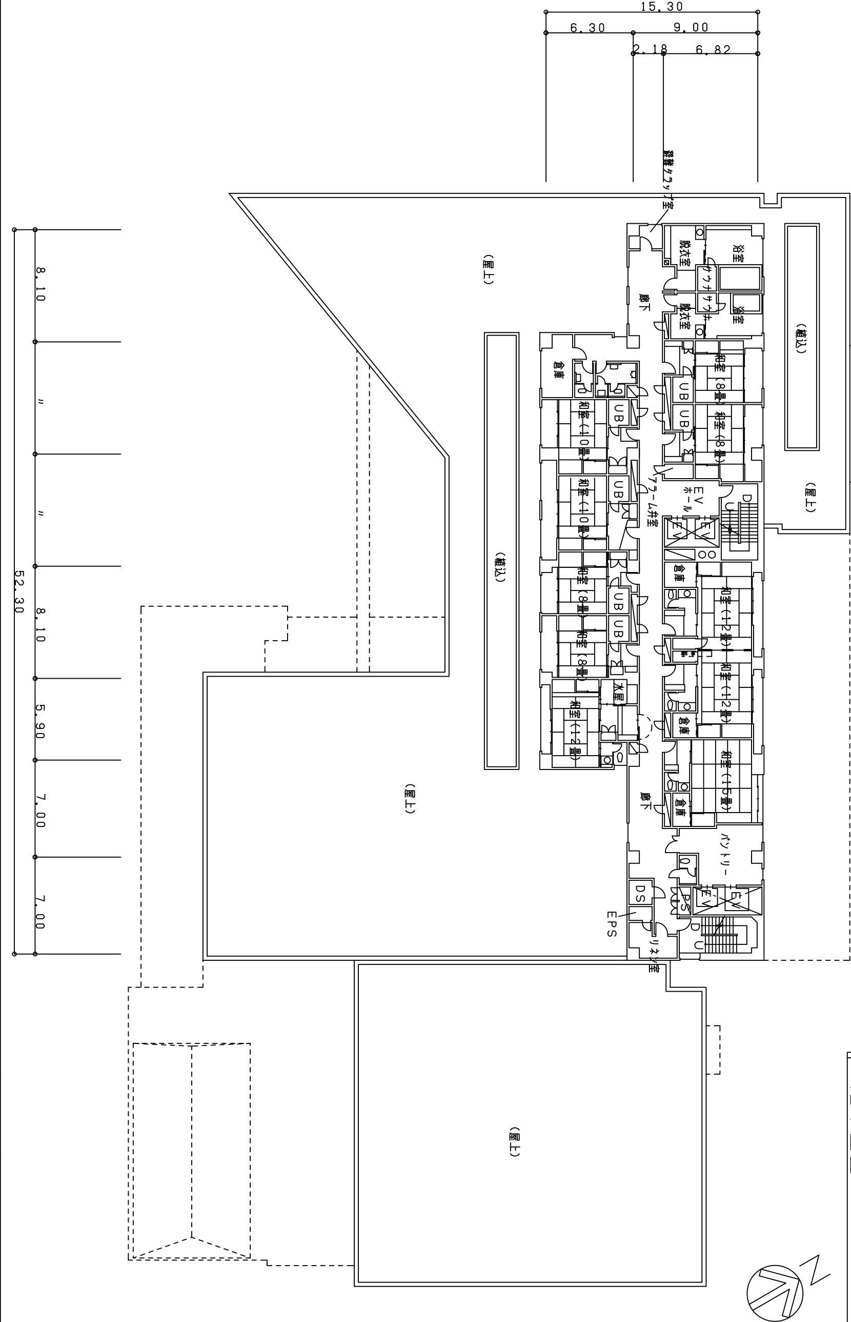
4階平面図 S:1/400
